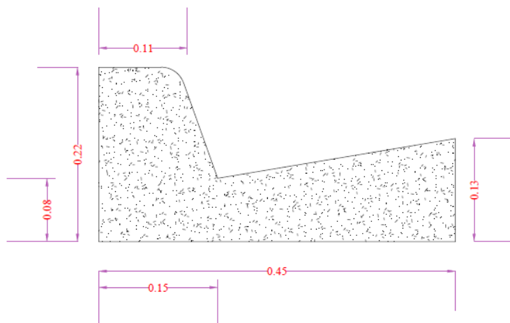
FIGURA 1- CORTE ESQUEMÁTICO DE GUIA E SARJETA CONJUGADA
