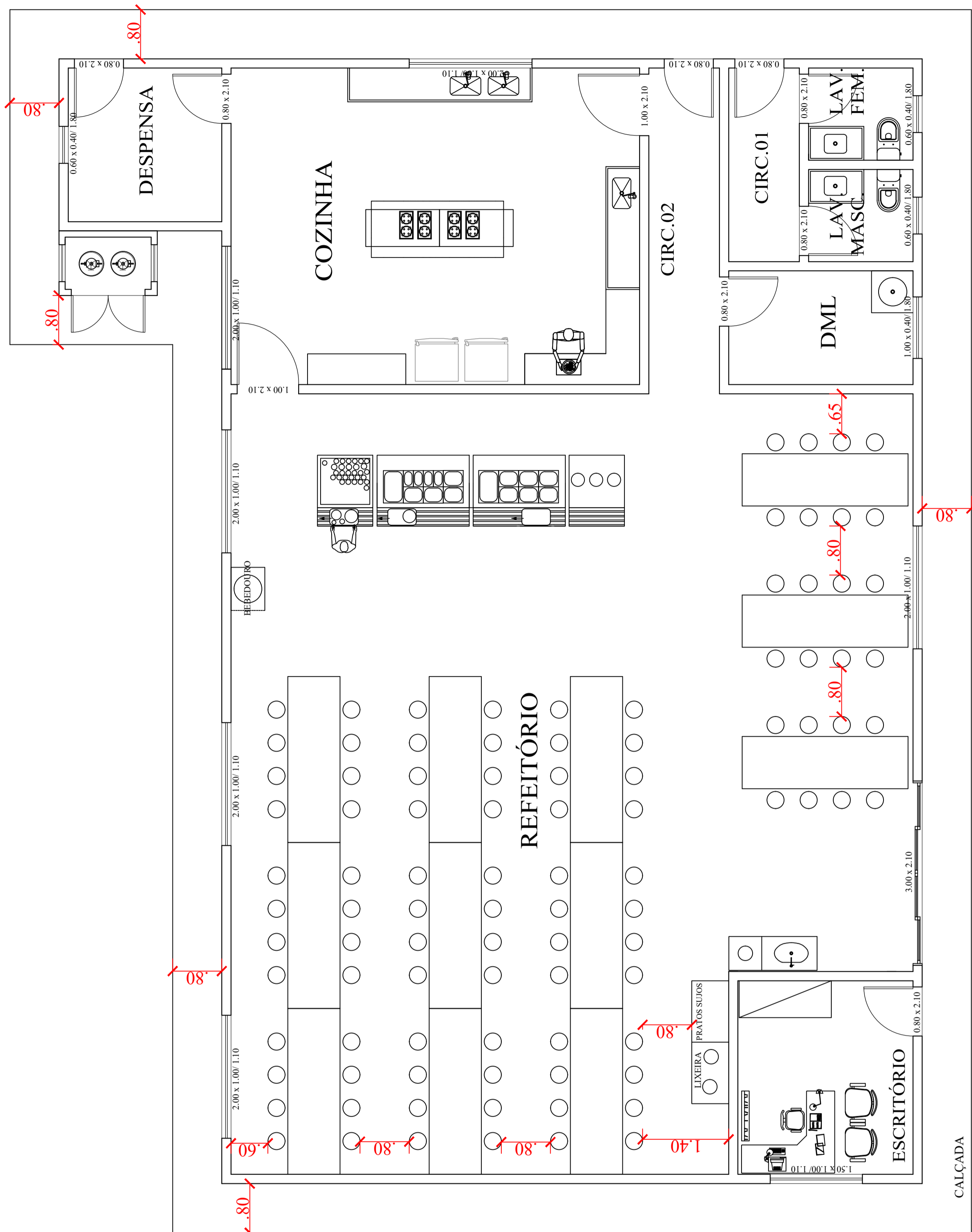
LAYOUT REFEITÓRIO ESCALA 1:50
